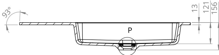
PRZEKRÓJ M-M SKALA 1 : 10
